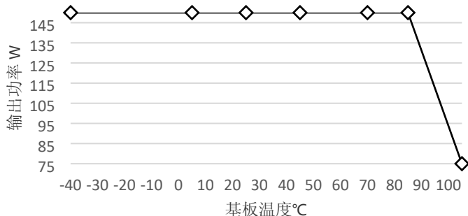
额定输入降额曲线图
