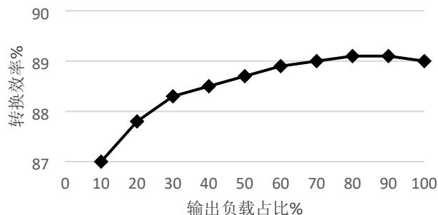
负载效率曲线
