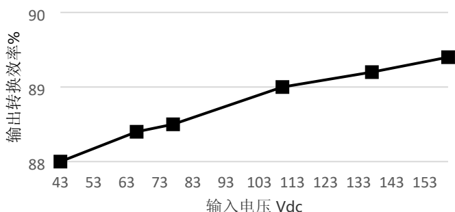
输入电压降额曲线
